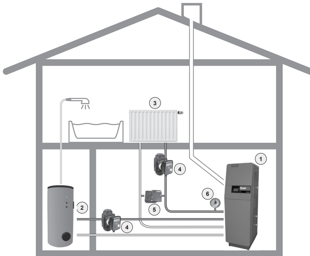
Exemple de système avec MultiJet® (12-25)
