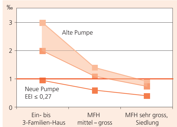
Verhältnis der elektrischen Pumpenleistung zur maximal benötigten thermischen Heizleistung (Norm-Heizlast \Phi_{th,n} ): Promille-Regel, 1‰ = 0,001. Für sehr kalte Klimazonen Verschiebung nach unten (ca. 1/3 weniger), für warme nach oben. Für Fussbodenheizungen bis zu 1/2 des Werts nach oben.
