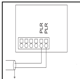
Fig. 4: PLR
