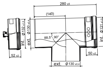
Pièce en T d'inspection E130 PP - 90° avec orifice de mesure
