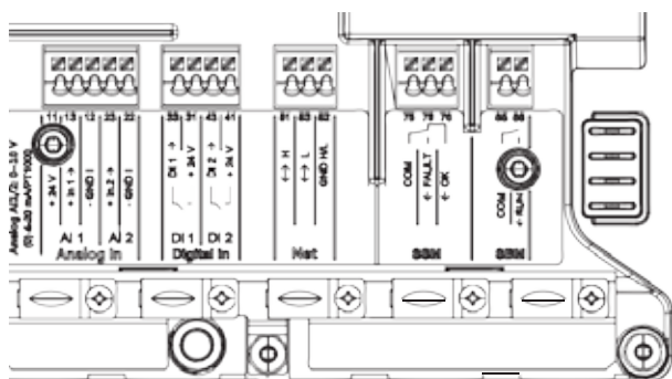
Bornier de la Stratos MAXO
