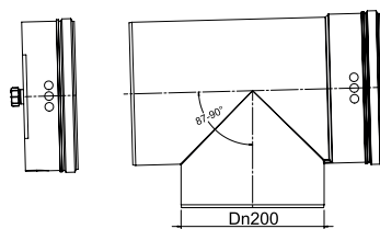
Pièce en T d'inspection E200 PP - 90° avec orifice de mesure
