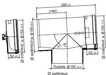
Pièce en T d'inspection E150 PP - 90° avec orifice de mesure L = 280 mm
