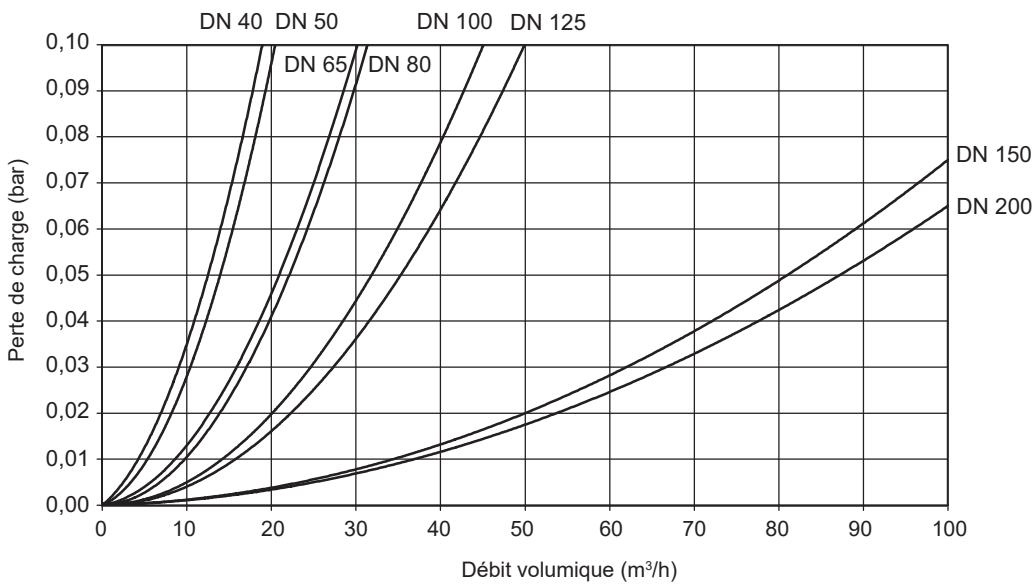
Courbe caractéristique de débit Séparateurs hydrauliques MH (40) à MH (200)
